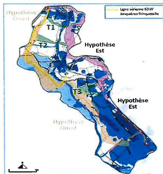
projet de tracé de la ligne aérienne haute tension
